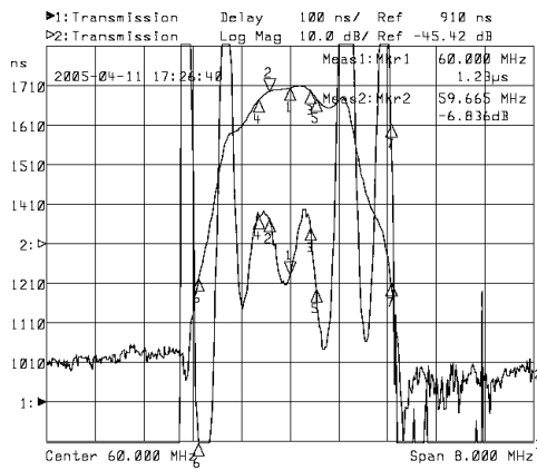
Horizontal: 0.8MHz/Div Vertical: 100ns/Div&10dB/Div
